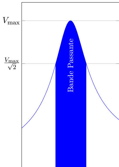
Bande passante
