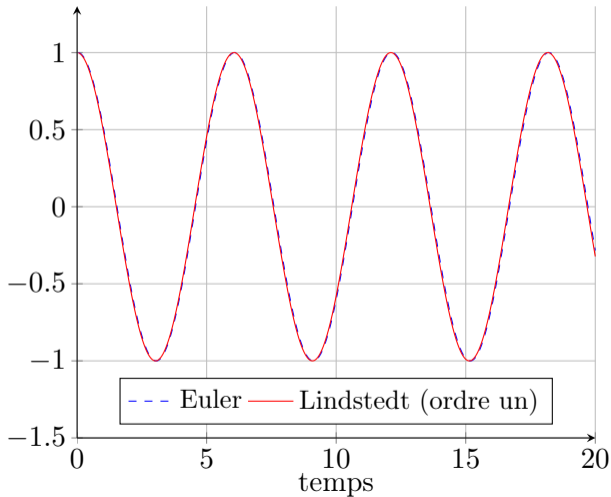
Oscillateur de Duffing : \epsilon = 0,1
