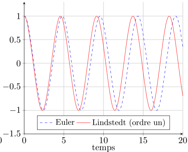
Oscillateur de Duffing : \epsilon = 1
